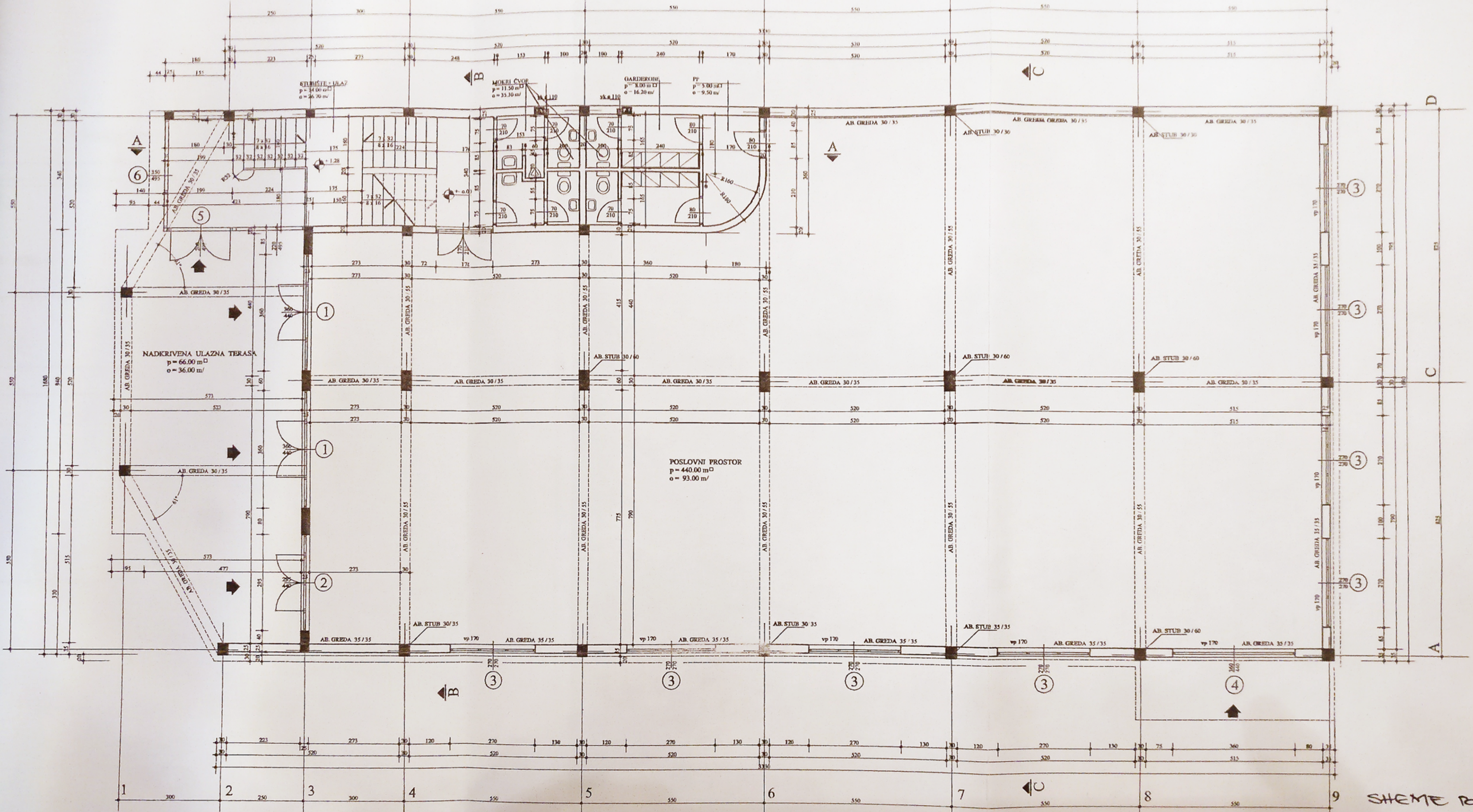
TLOCRT II mj. 1 : 50 prizemlje
